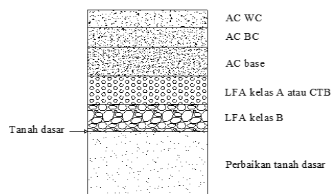
Gambar 1. Susunan perkerasan lentur pada tanah asli (Bina Marga, 2017)
