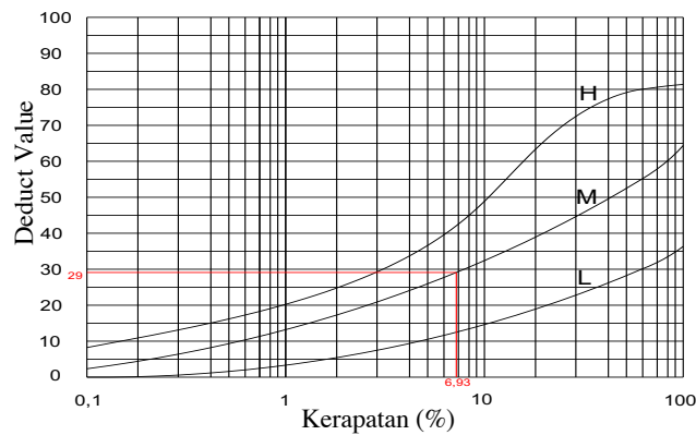
Gambar 4. Grafik kerusakan retak (ASTM internasional, 2007)
