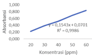
Gambar 1. Hasil linieritas asam galat
