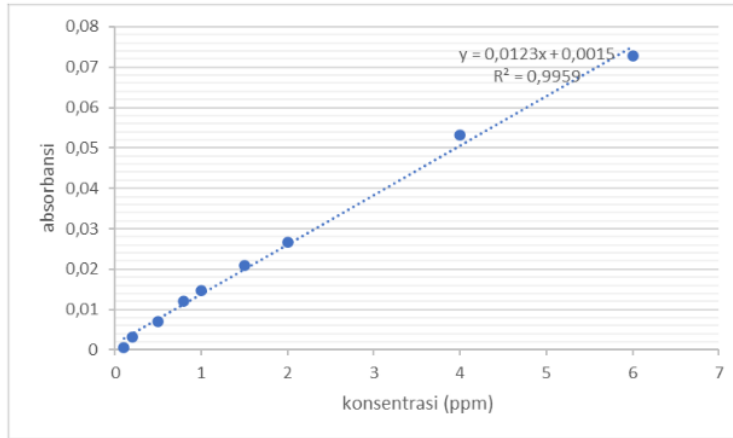
Gambar 2. Grafik regresi linier standar Fe
