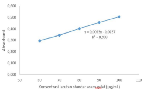
Gambar 2. Kurva kalibrasi asam galat
