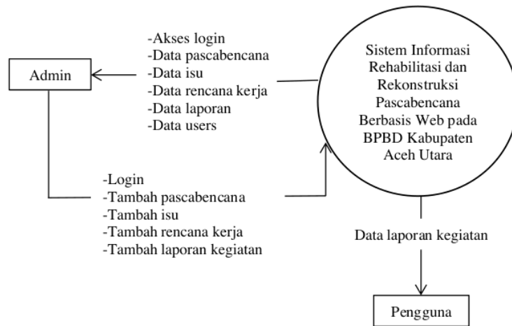
Gambar 1. Diagram Konteks
