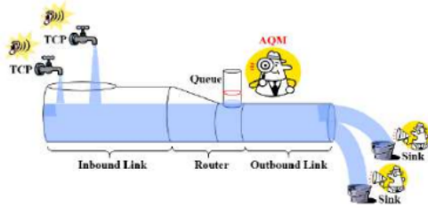
Gambar 3. Mekanisme AQM
