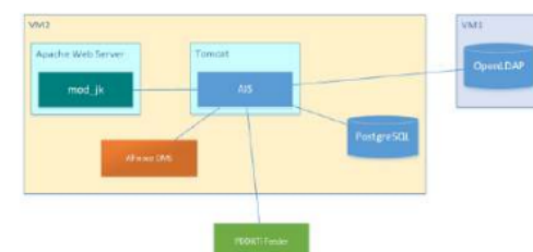
Gambar 13. Rancangan alokasi LDAP pada VMWare 1
