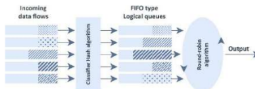
Gambar 2. Mekanisme SFQ
