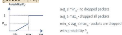
Gambar 1 Skema Algoritma RED
